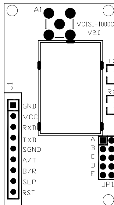
图 1.引脚位置图
