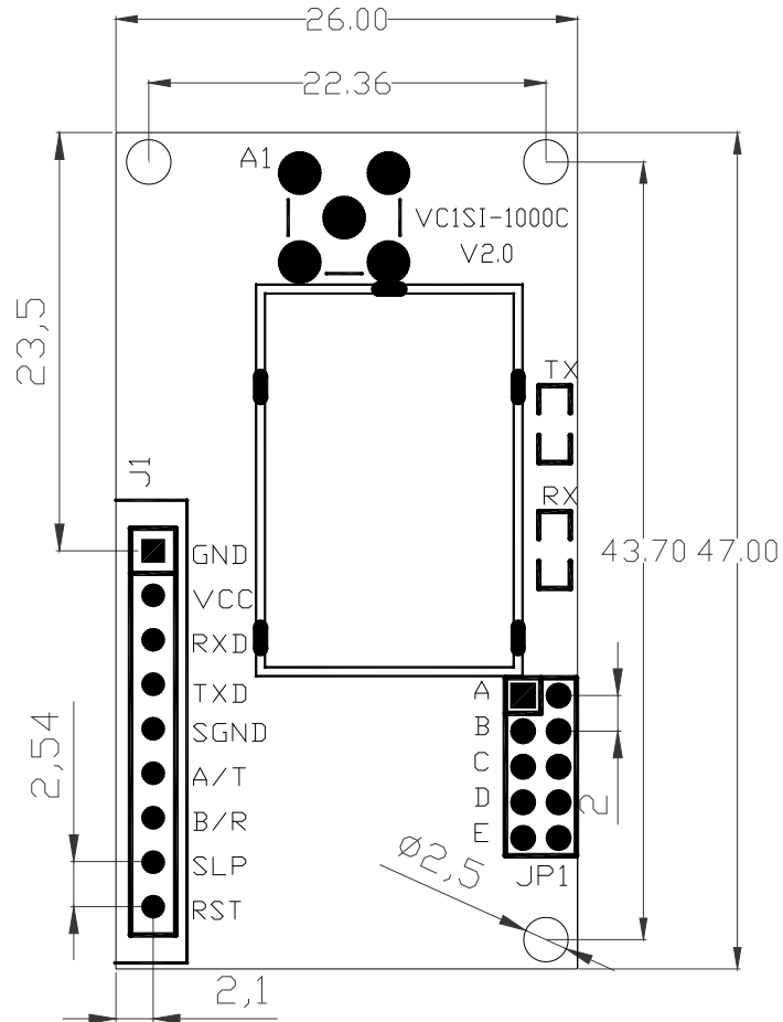
图 2.产品尺寸图
